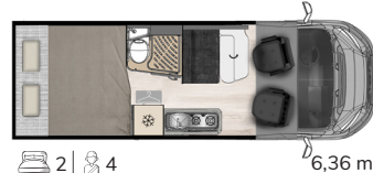
Menfys S-Line/ Prestige 4 Maxi
