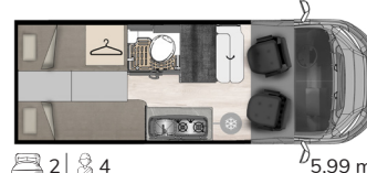
Menfys S-Line/ Prestige 4 CS
